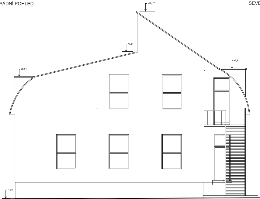
ZÁPADNÍ POHLED
