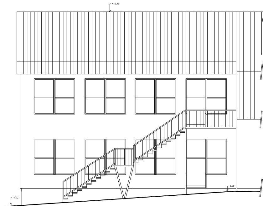
JIŽNÍ POHLED
